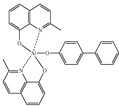
BAlq
